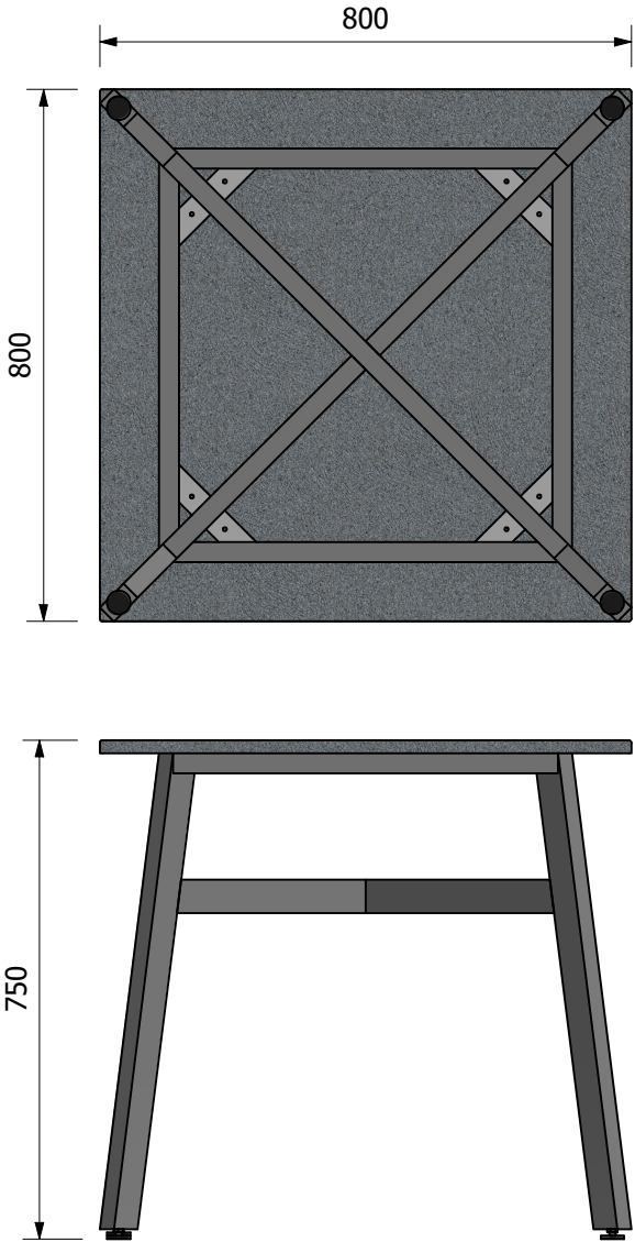
Dimensiones generales
