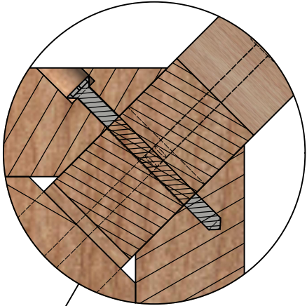
FN ( 1 : 2 )
