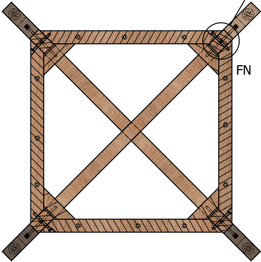
FJ-FJ ( 0.085 )
