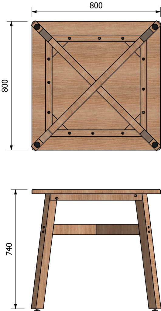
Dimensiones generales
