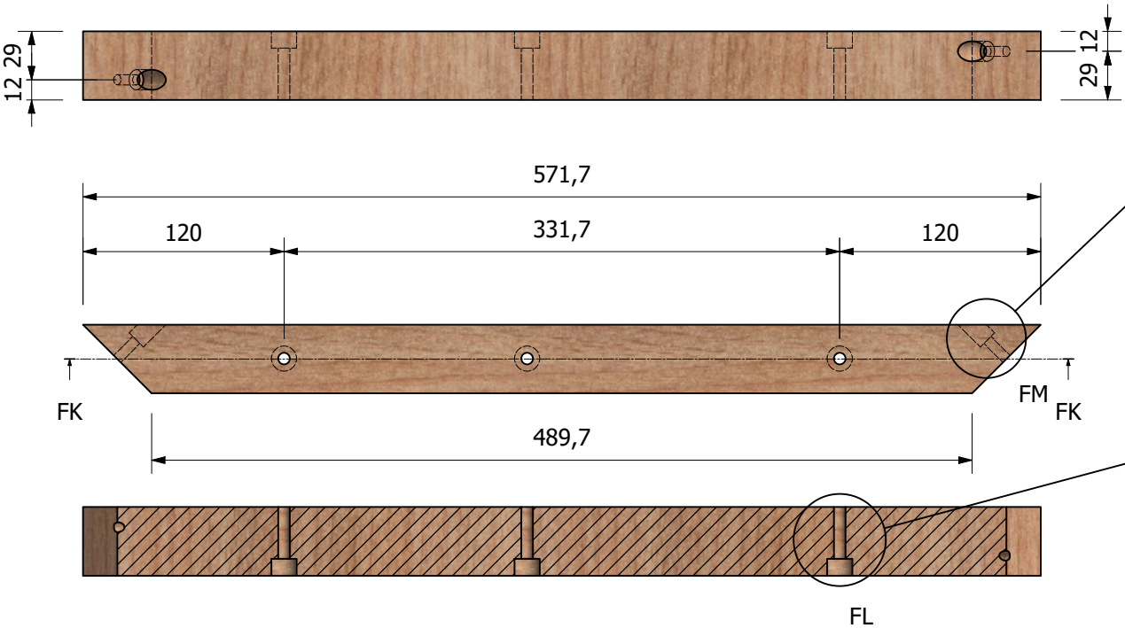
FK-FK ( 1 : 4 )
