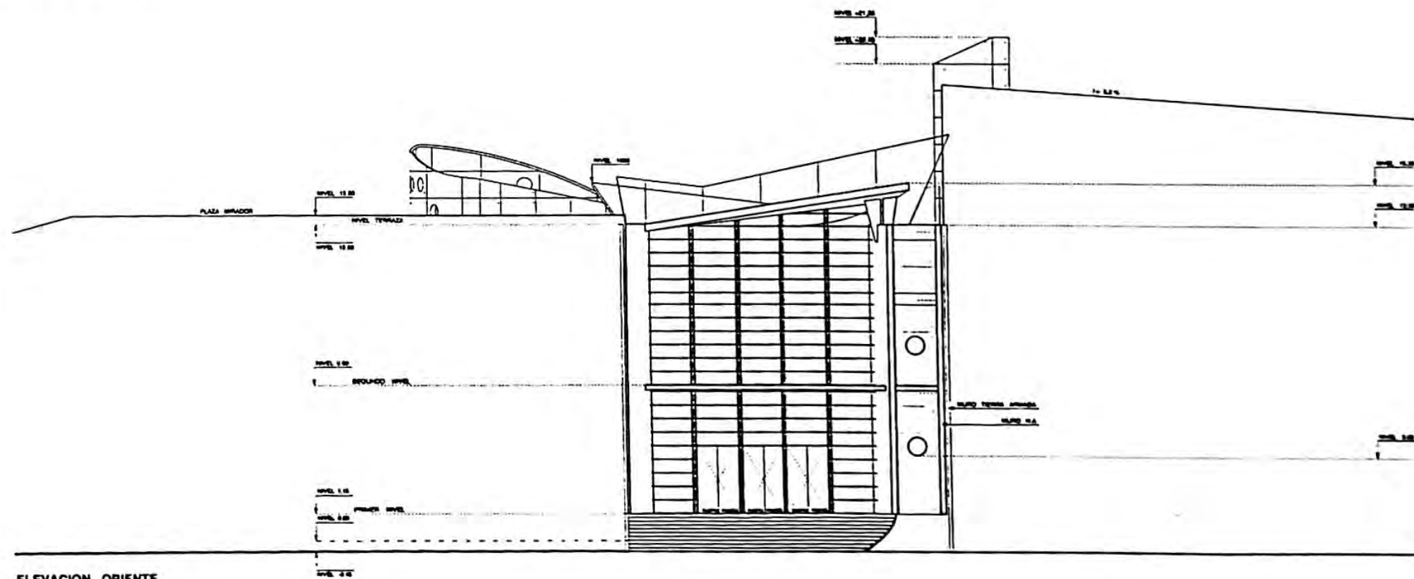
ELEVACION ORIENTE TUNEL DEL TIEMPO ESCALA 1/20
