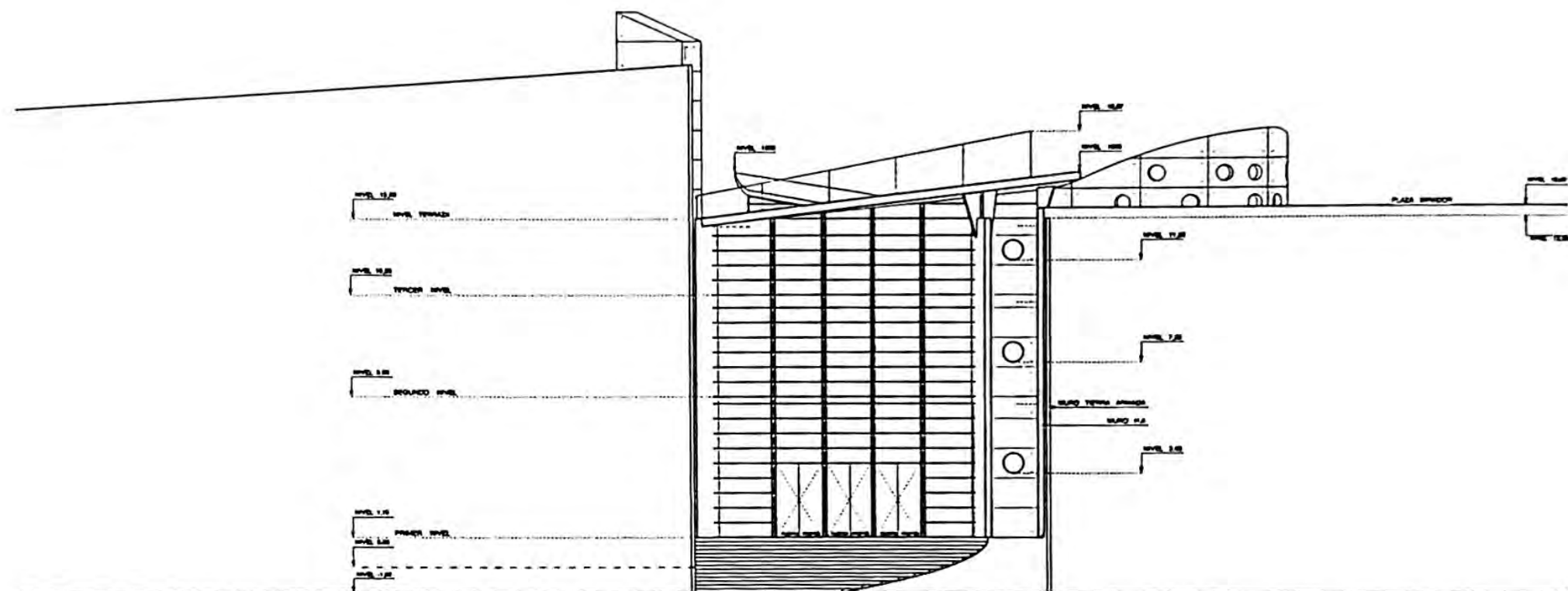
ELEVACION PONIENTE TUNEL DEL TIEMPO ESCALA 1/20
